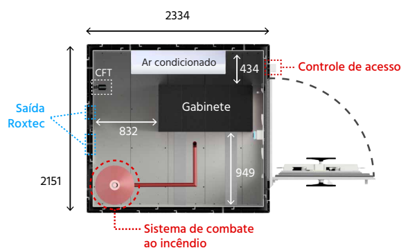
Layout Rack seguro para 1 gabinete - Montado in loco
