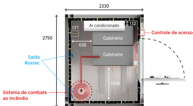
Layout Rack seguro para 2 gabinetes - içável
